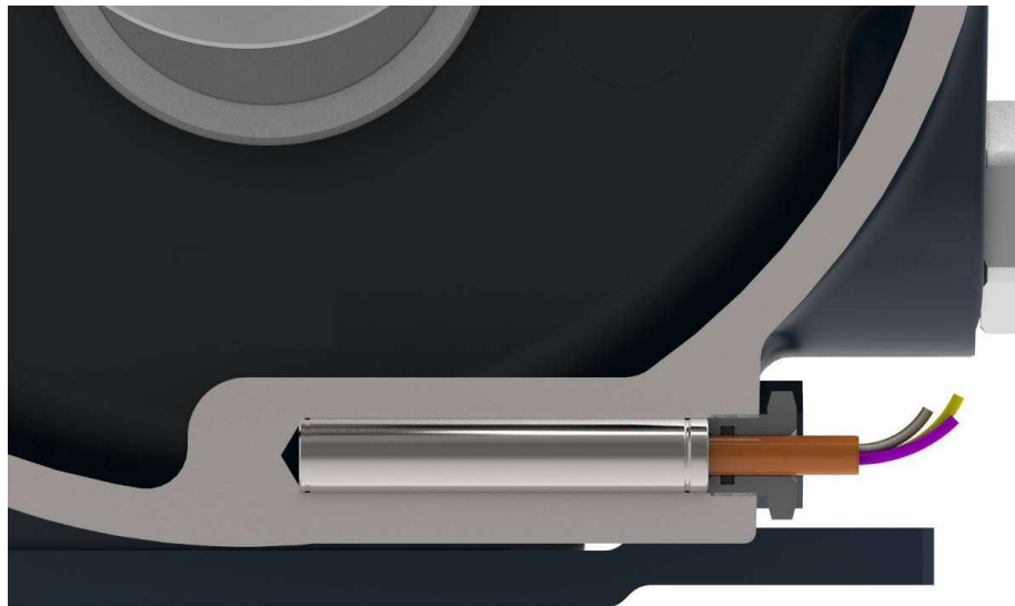
Resistenza carter installata nel apposito foro sul carter / Crankcase heater installed in the housing bore / Résistance de carter installé dans l'alésage du logement / Ölumpfheizung in der Gehäusebohrung installiert
