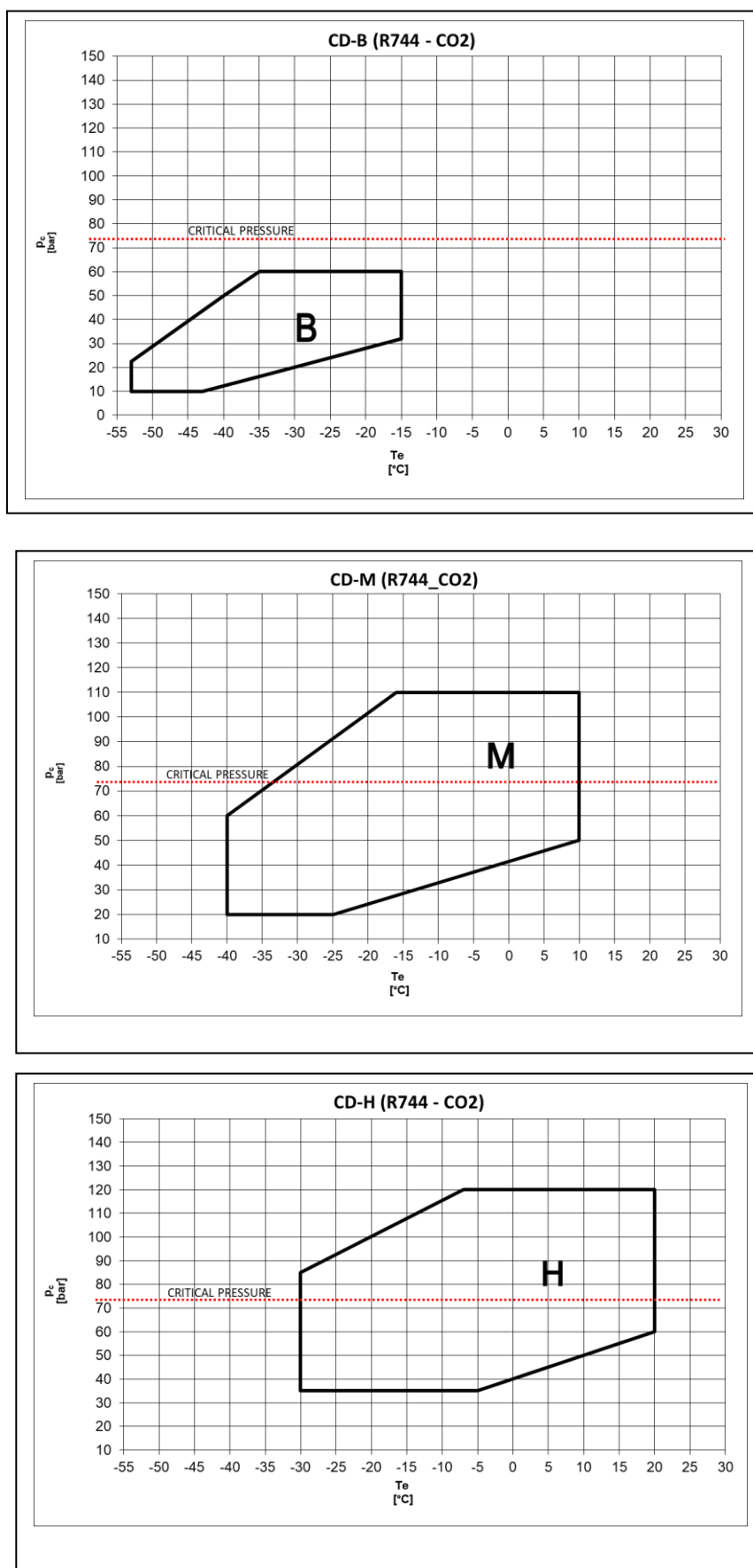
Fig. 4: CD600 - Limiti d'applicazione – Application limits – Champs d'application
